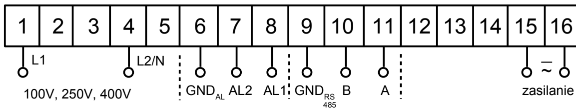
Rys. 4. Połączenia elektryczne miernika N20ZPLUS z pomiarem napięcia i częstotliwości
