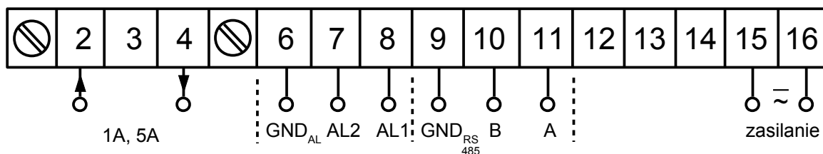
Rys. 5. Połączenia elektryczne miernika N20ZPLUS z pomiarem prądu
