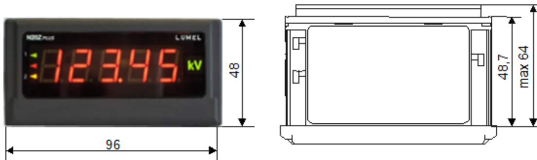
Rys. 3. Gabaryty miernika
